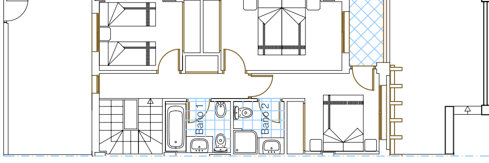
Planta Primera
