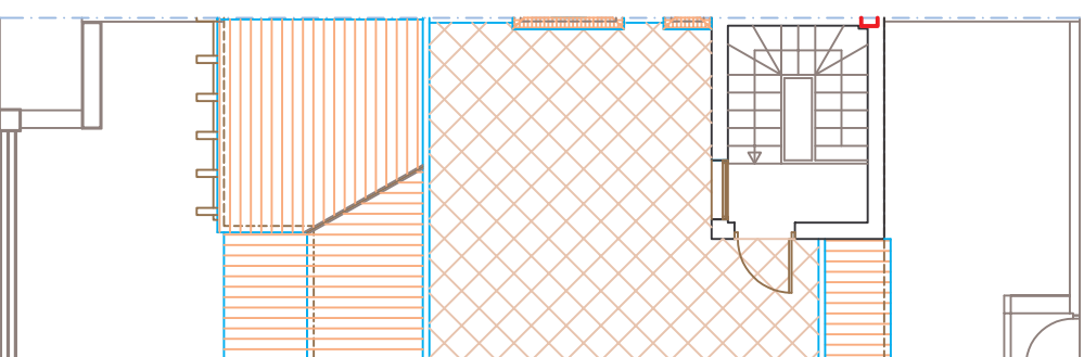
Planta Solarium
