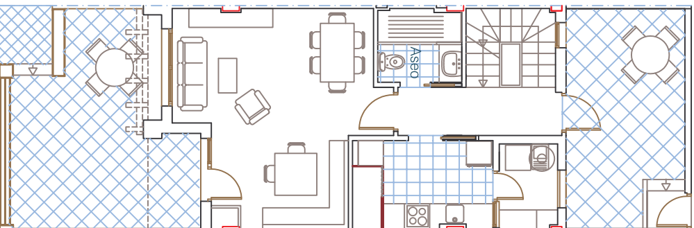
Planta Baja
