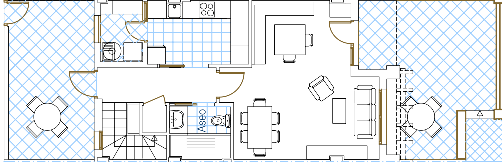
Planta Baja
