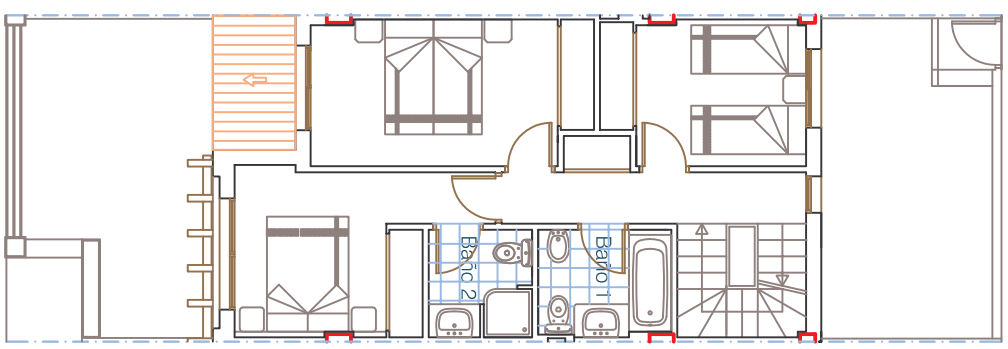
Planta Primera
